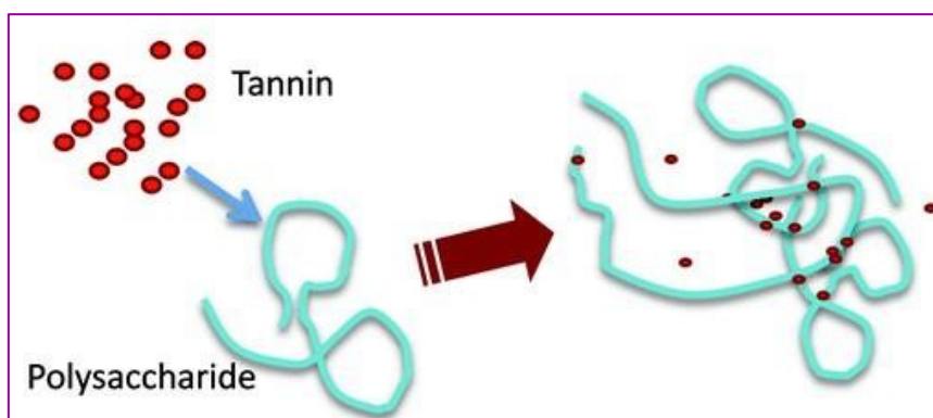
Σχήμα 1: Επικάλυψη στυπτικών ταννινών από πολυσακχαρίτες που προέρχονται από κυτταρικά τοιχώματα σακχαρομυκήτων.
